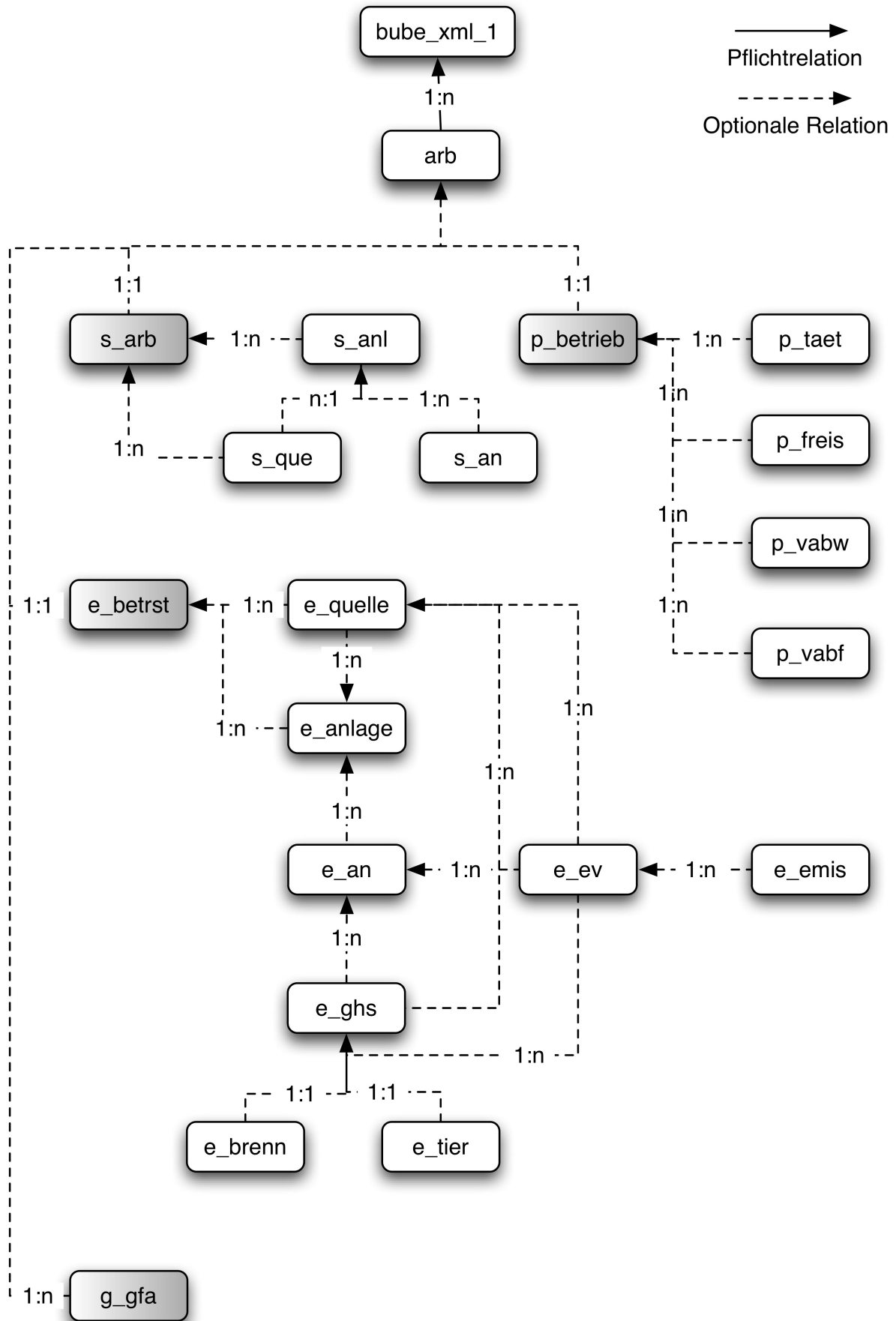
Abbildung 1: Datenmodell
