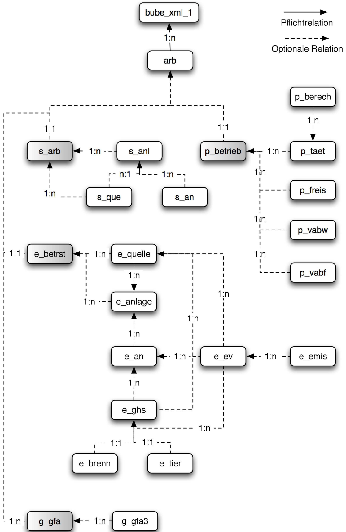
Abbildung 1: Datenmodell
