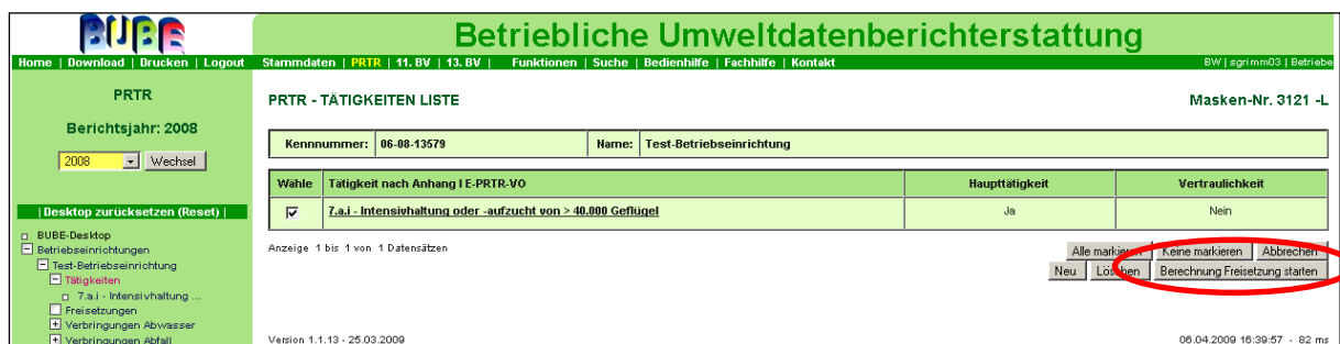
Abbildung 43: Berechnungsvorgang starten
